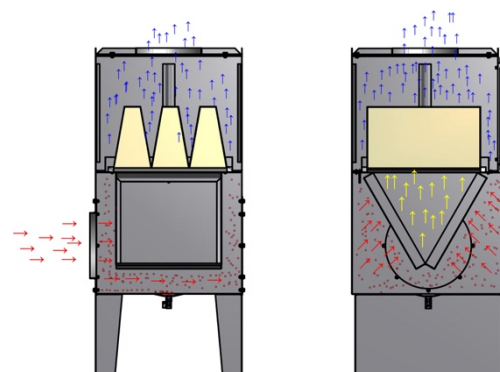
OUK met opgebouwde M7 ventilatormodule
